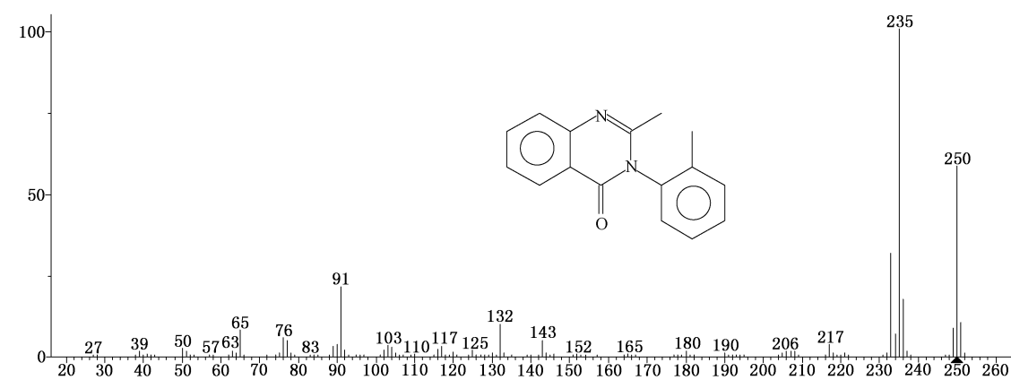
图 B.2 安眠酮质谱图
