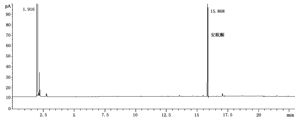
图 B.1 安眠酮气相色谱图
